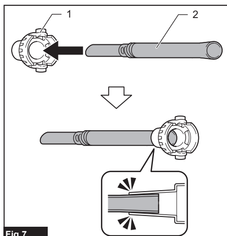
► 1. Buse 13 2. Buse longue R
