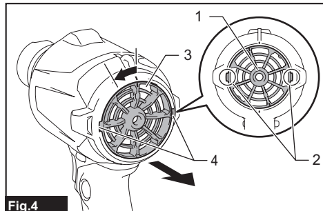
► 1. Capuchon antipoussière 2. Languettes de verrouillage 3. Entrée d'aspiration 4. Rainures de guidage
