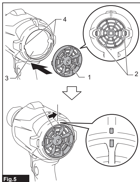
► 1. Capuchon antipoussière 2. Languettes de verrouillage 3. Entrée d'aspiration 4. Rainures de guidage
